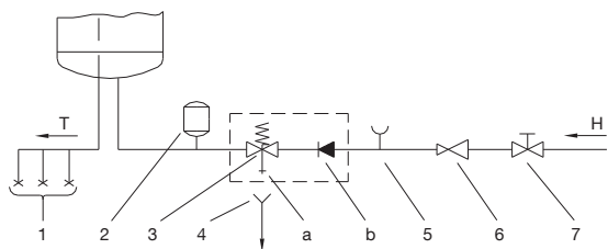
SI. 2: Zatvoreni sistem (pod pritiskom)
