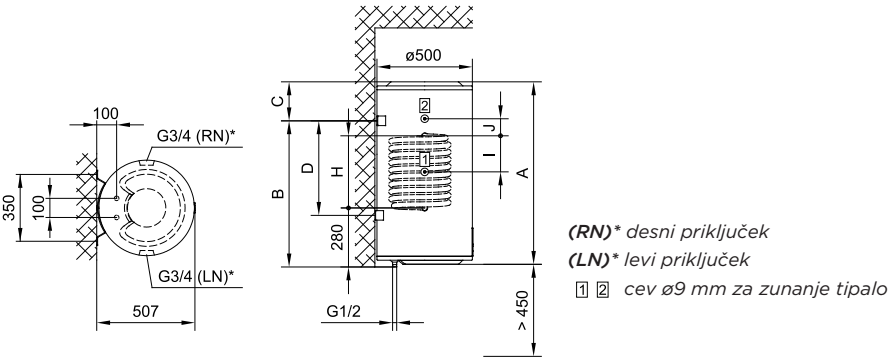
Sl. 1: Pokončna namestitev na steno
