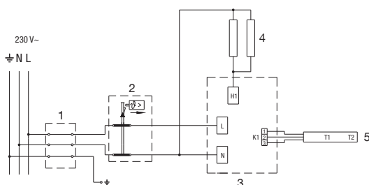
Сл. 6: Шема на електрично поврзување
