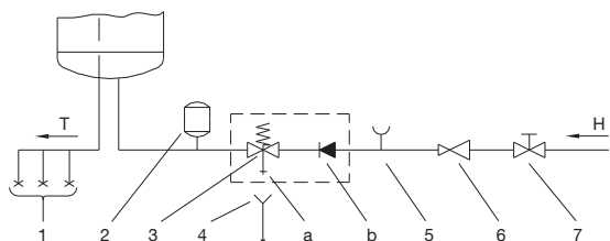
Сл. 2: Затворен систем (со притисок)
