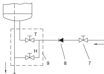
Bild 3: Offenes System (druckloses System)
