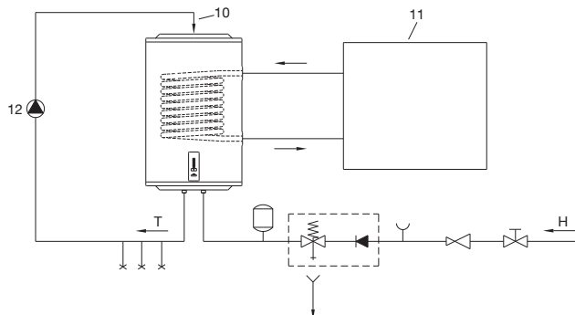
SI. 4: Priklop grelnika na dodatni energetski vir
