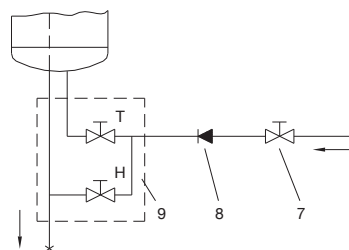
Fig. 3: Sistemi i hapur (pa presion)
