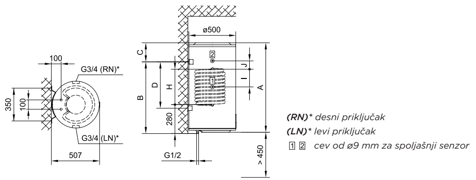
Sl. 1: Vertikalno montiranje na zid
