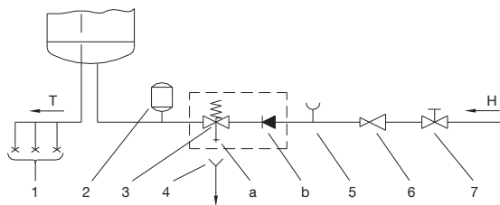
Bild 2: Geschlossenes System (druckfestes System)
