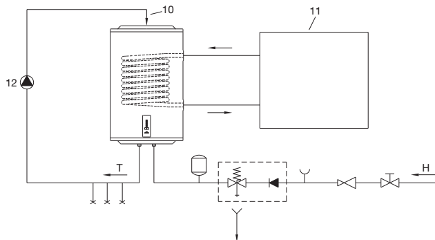
Fig. 4: Lidhja me burime tjera për ngrohje
