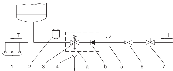
Fig. 2: Sistemi i mbyllur (me presion)
