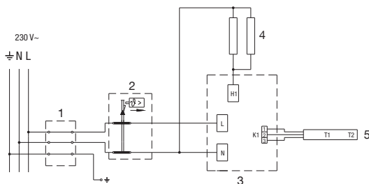
Bild 6: Elektroschaltbild
