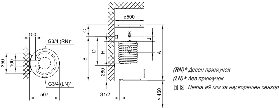
Сл. 1: Исправено поставување на сид
