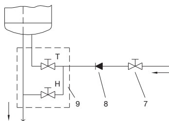
Сл. 3: Отворен систем (прелевен)
