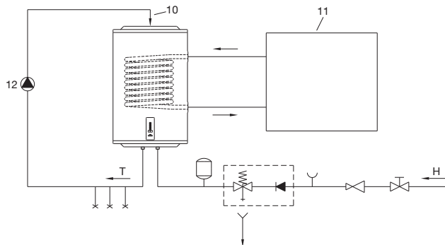
SI. 4: Priključivanje na druge izvore grejanja
