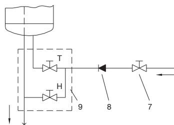
SI. 3: Odprti (netlačni) sistem
