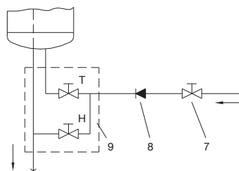
Sl. 3: Otvoreni (protočni) sustav
