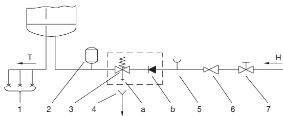
Sl. 2: Zatvoreni (tlačni) sustav
