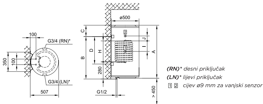
Sl. 1: Uspravno postavljanje na zid
