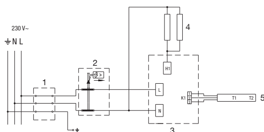
Sl. 6: Električna spojna shema
