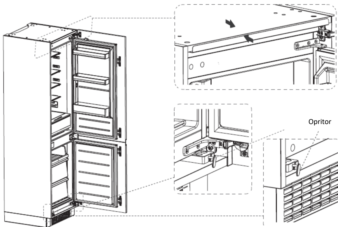
Marginea îndoită a pragului superior
