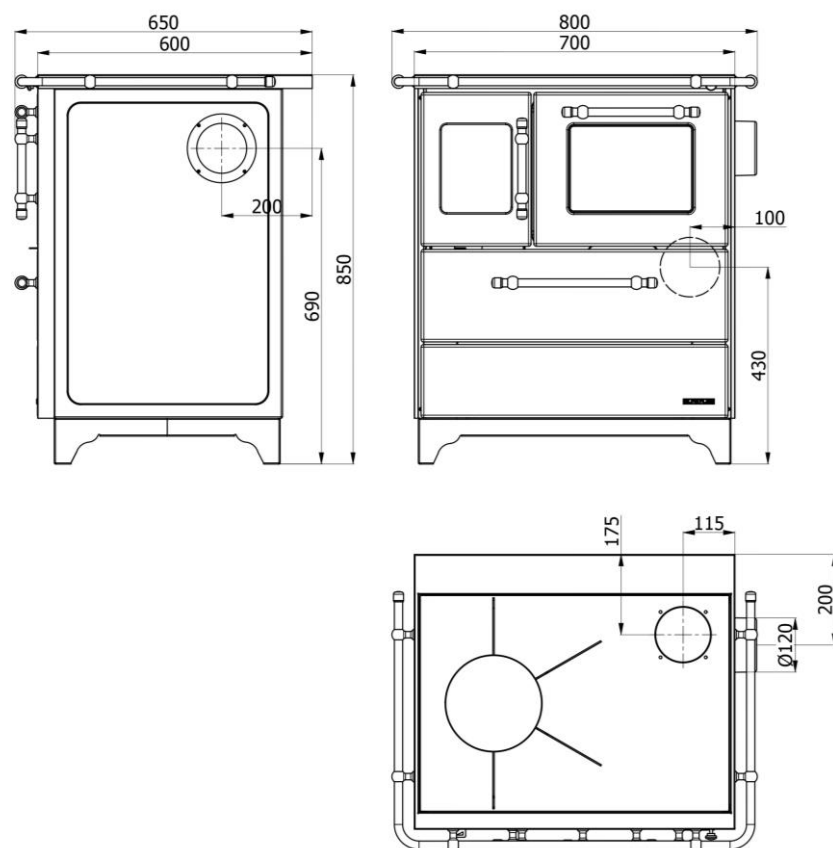
Slika 4 - DONNA70 - Dimenzije
