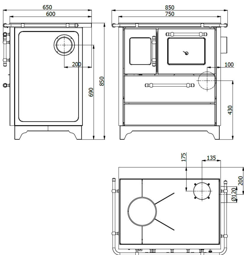
Slika 5 - DONNA 75- Dimenzije
