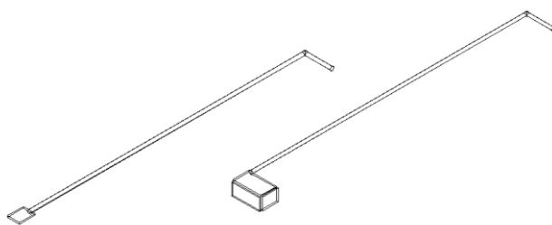
Slika 8. Pribor za čišćenje kotla
