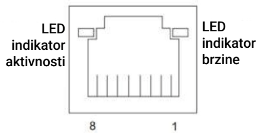
Slika 13. Priključak RJ45 (strana na kojoj je priključak)
