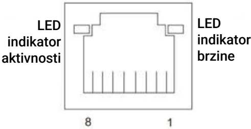
Slika 13. Priključak RJ45 (strana na kojoj je priključak)
