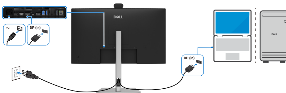
Slika 31. Priključivanje DisplayPort kabela
