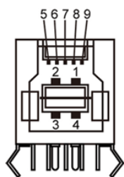
Slika 10. USB Type-B 5 Gbps dolazni priključak
