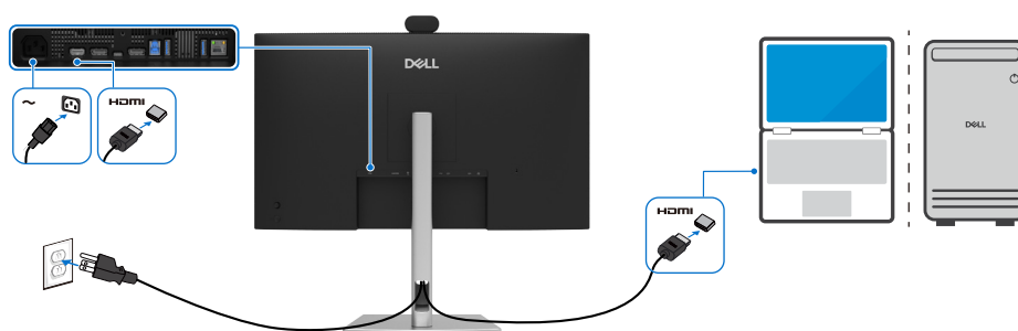
Slika 30. Priključivanje HDMI kabla
