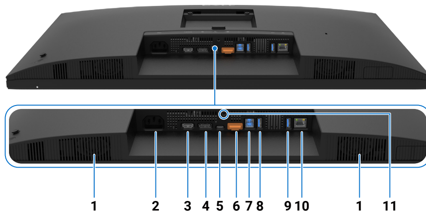
Slika 3. Pogled na monitor odozdo
