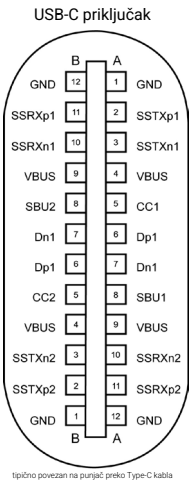
Slika 9. USB-C priključak
