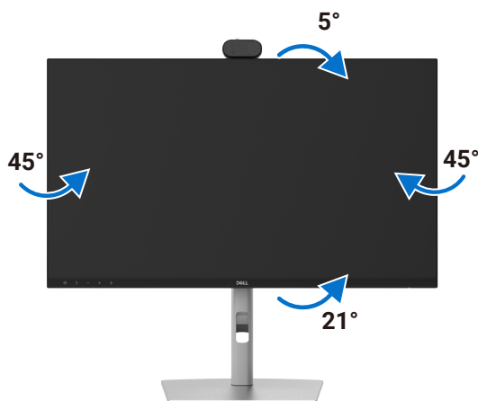
Slika 25. Podešavanje nagiba i obrtanja oko svoje ose (P2426HEB/P2726DEB).
