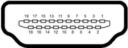
Slika 8. HDMI priključak
