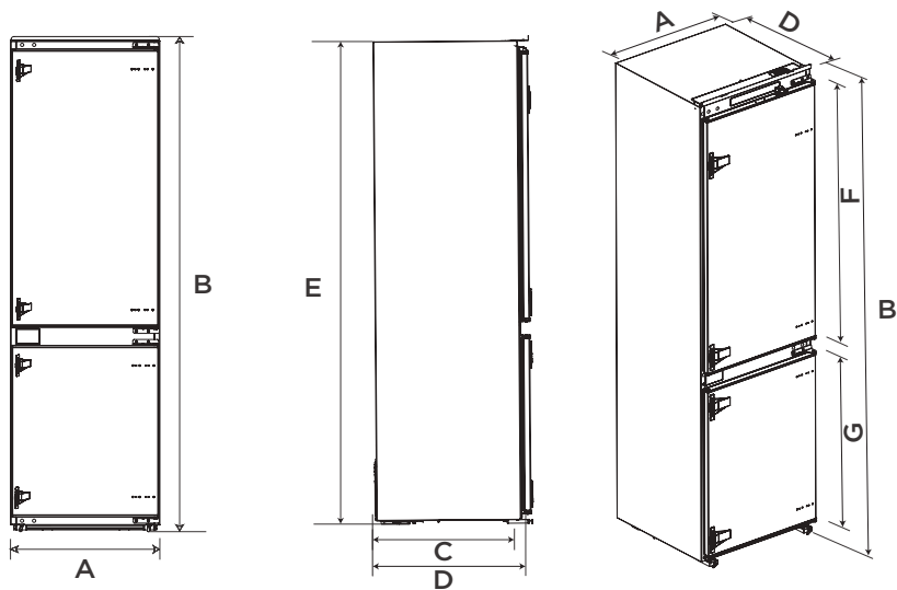
Diagrama spațiului necesar (când ușa este deschisă și când ușa este închisă)
