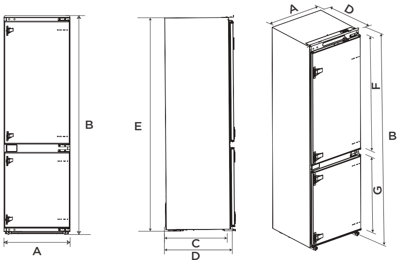
Диаграма на пространствените изисквания (при отворена и при затворена врата)
