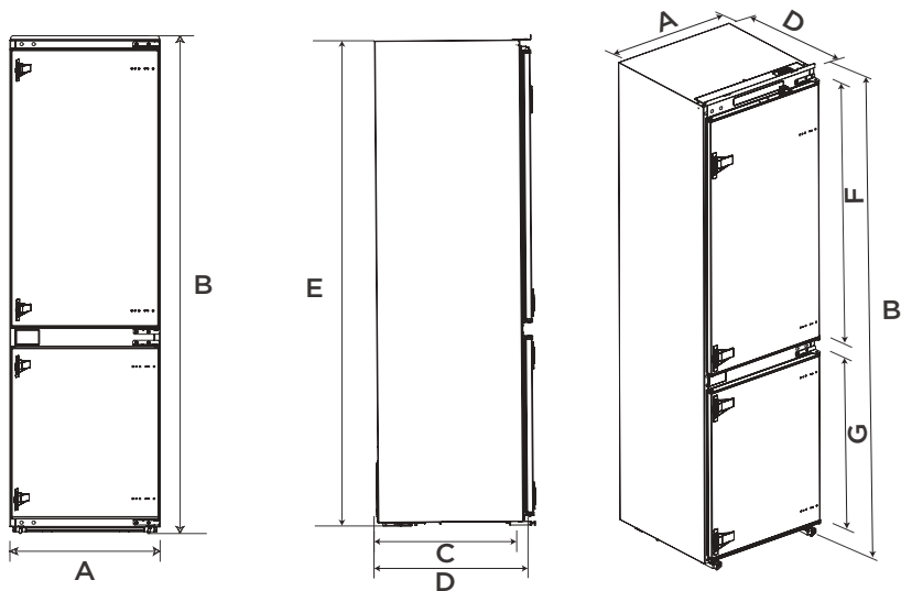
Schéma požadavků na prostor (při otevřených a zavřených dveřích)
