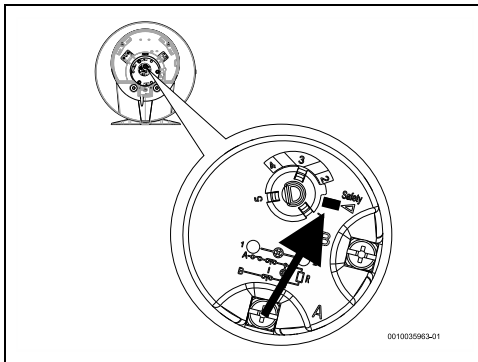
Rys. 30 Termostat bezpieczeństwa (modele bez pokrętki nastawczego temperatury)
