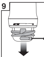
Rimuovere la ventola compattatrice con l'apposito magnete
