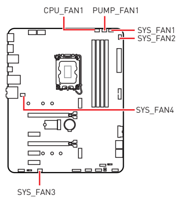
风扇接口规格
