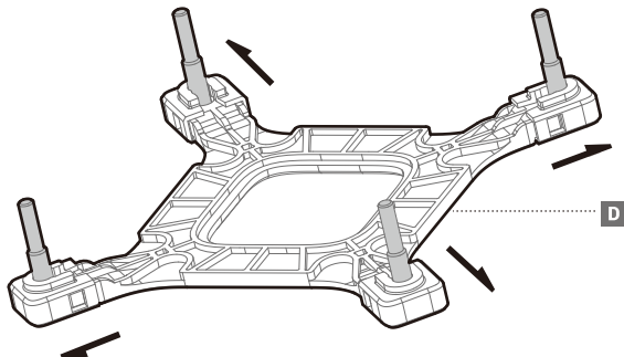
LGA1700
