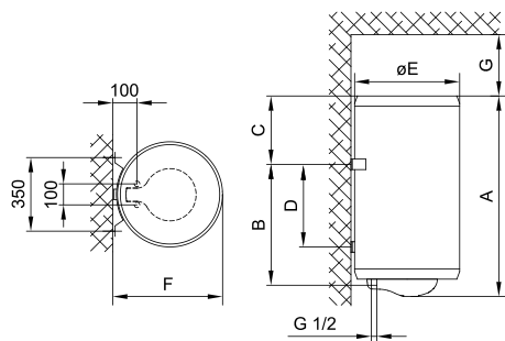
Anschluss- und Montagedimensionen des Warmwasserbereiters [mm]
