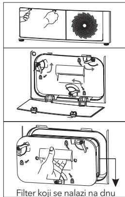
Filter koji se nalazi na dnu mašine
