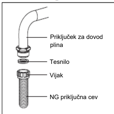
NG konektor
