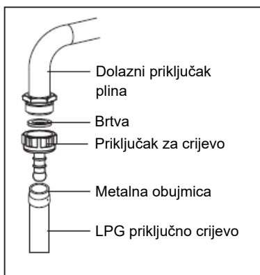
LPG priključenje
