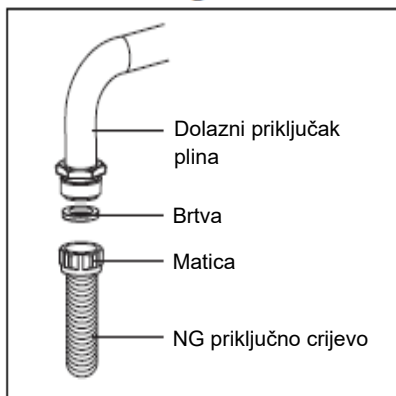
NG priključenje
