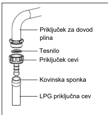
LPG konektor
