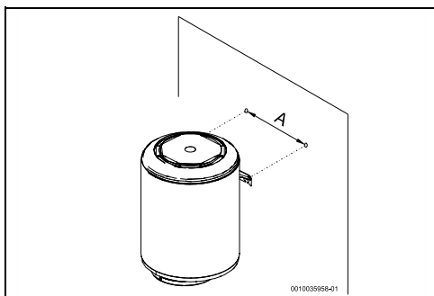
sl. 10 Vertikalna instalacija (zidna montaža)
