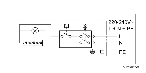
fig. 17 Skema e lidhjes
