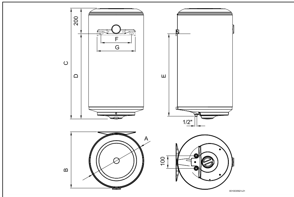
2. ábra Méretek mm-ben (falra szerelés, fügőleges szerelés)
