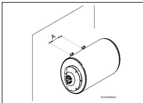
Сл. 11 Хоризонтална инсталација (монтажа на сид, TR1000...H)
