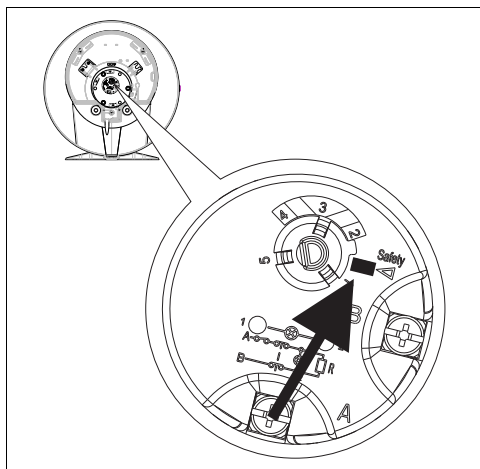
Sl.15 Sigurnosni termostaat (Tronic 1000T)
