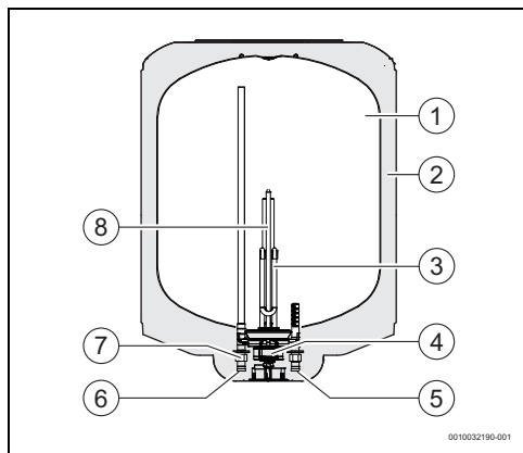
Rys. 4 Komponenty urządzenia
