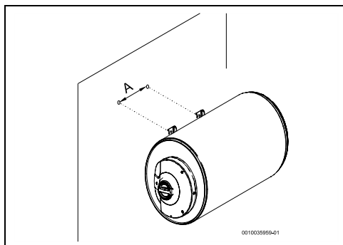
Rys. 11 Montaż poziomy (montaż na ścianie TR1000...H)
